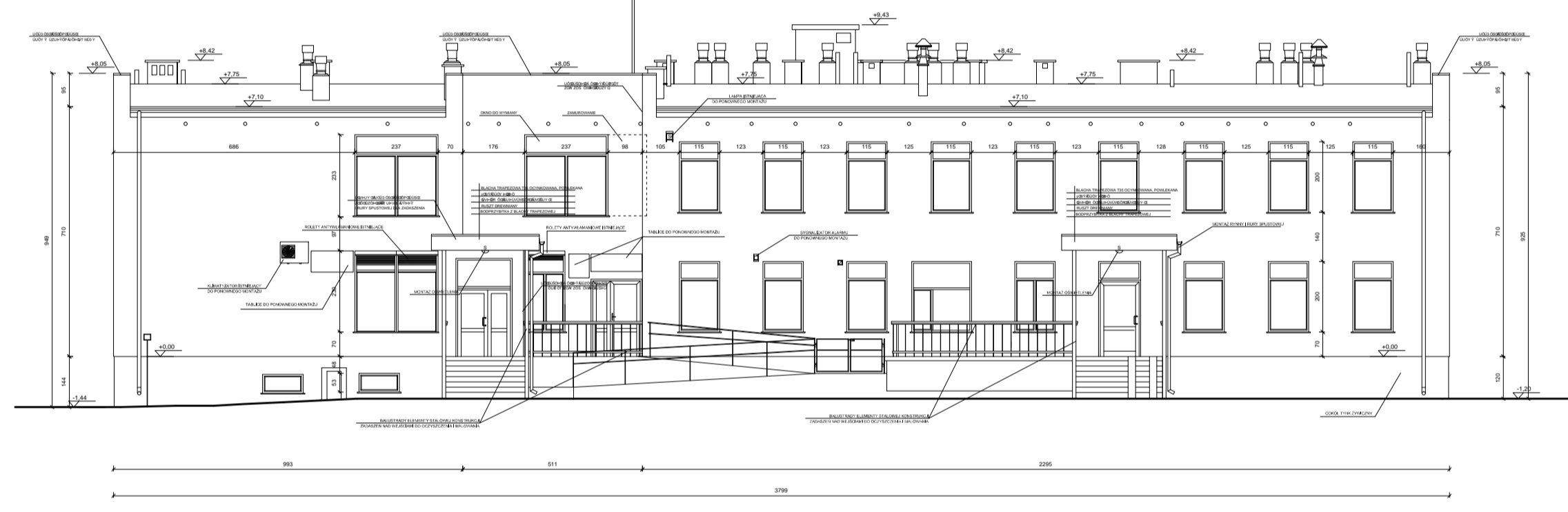
ELEWACJA PÓŁNOCNA
