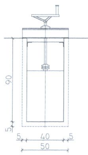
SCHEMAT WYKONANIA OSADZENIE ZASUW S
