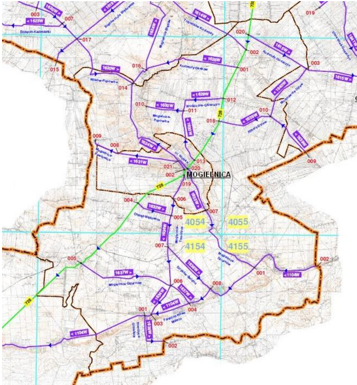
Ryc. 22: Model sieci dróg powiatowych oraz przebieg drogi krajowej nr 728 w gminie - źródło Powiatowy Zarząd Dróg Grójec
