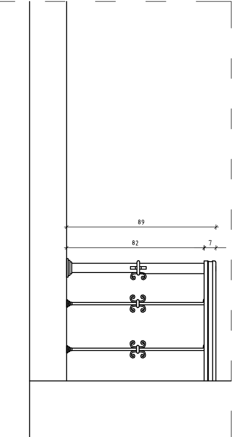
WIDOK SPOCZNIKA NA KOŃCU BIEGU SCHODÓW
