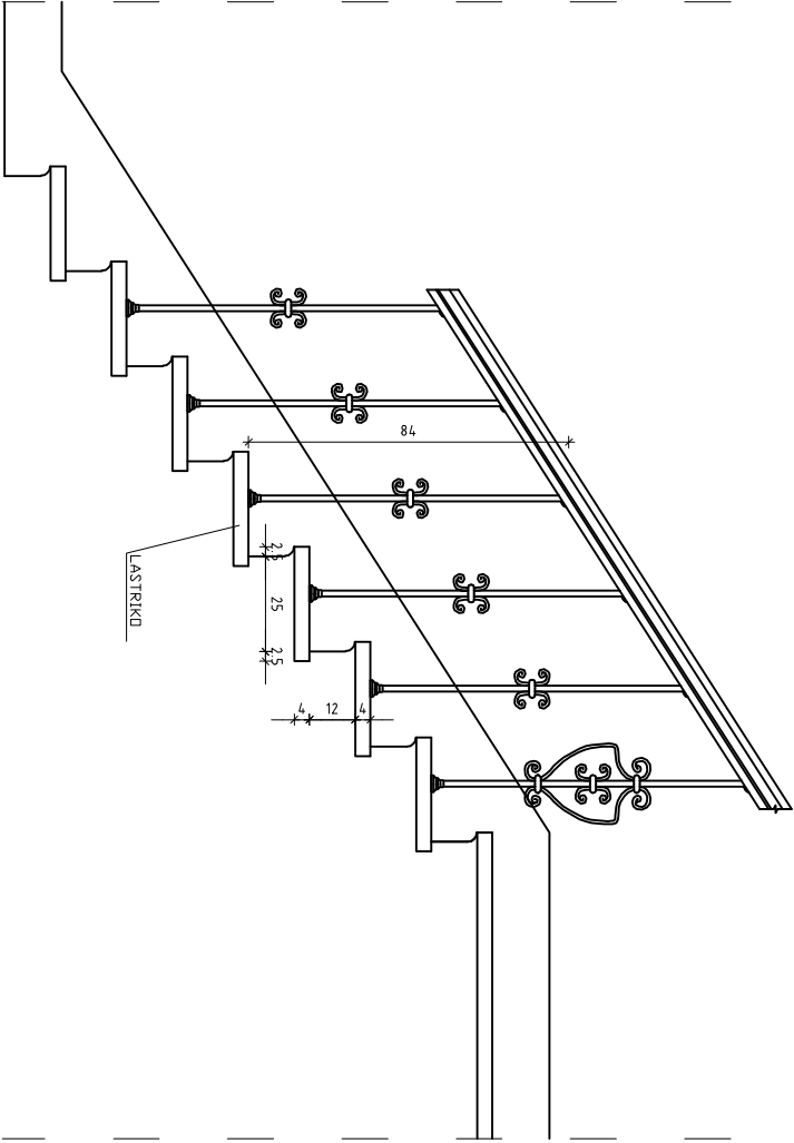
WIDOK 1. BIEGU SCHODÓW
